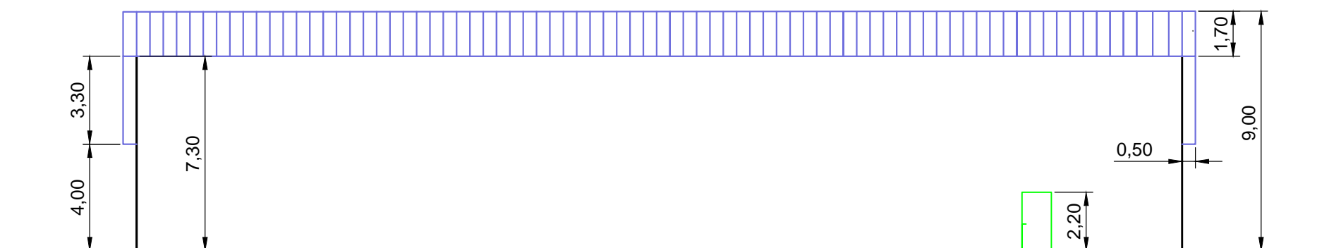
Façade nord
