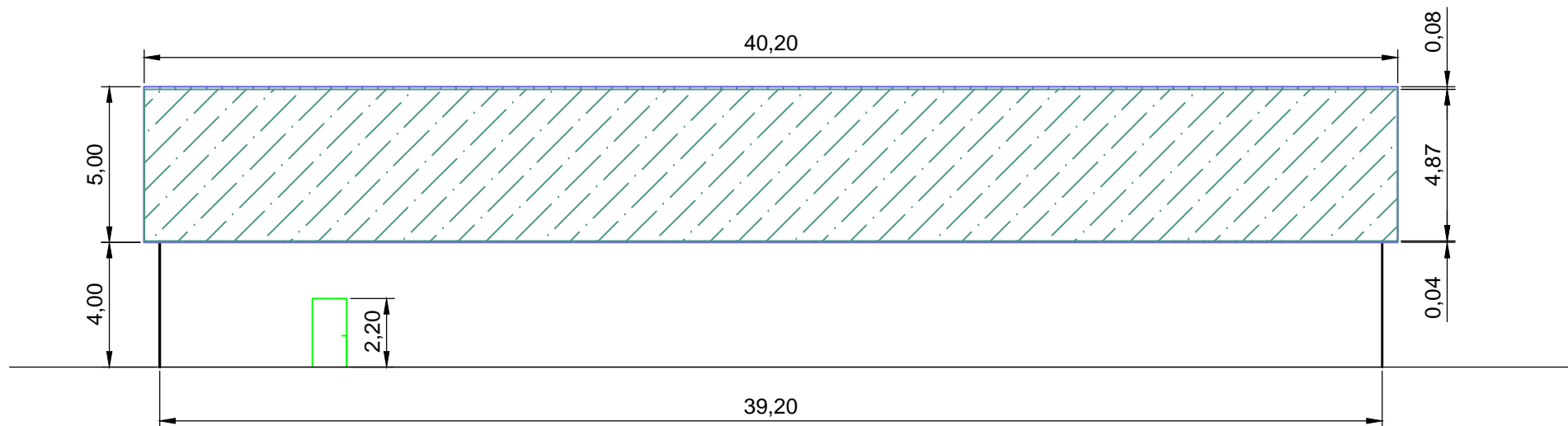
Façade sud
